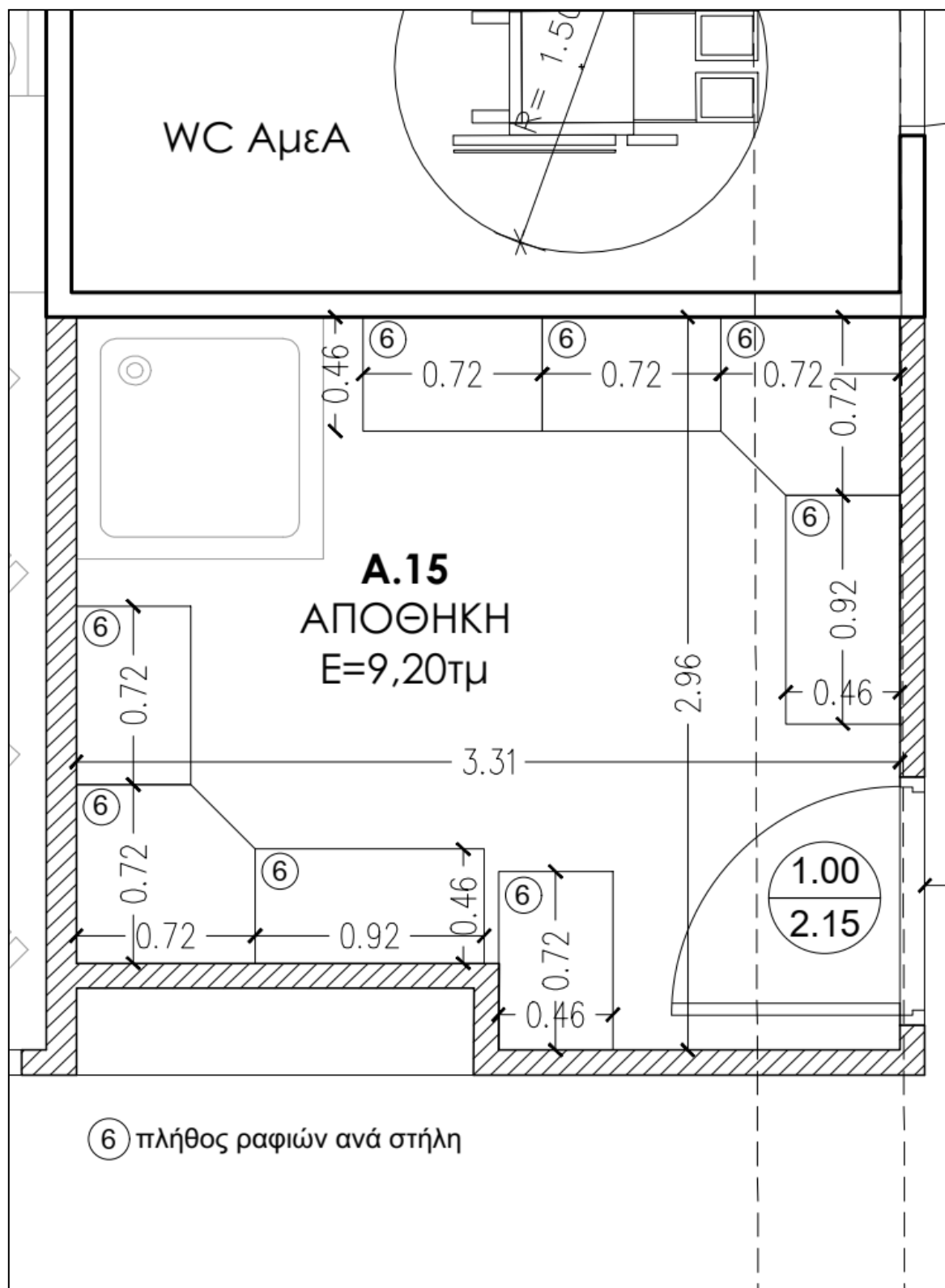
Εικόνα 1. Διάταξη συστήματος ραφιών τύπου dexion σε αποθηκευτικό χώρο του 1 ου ορόφου.
