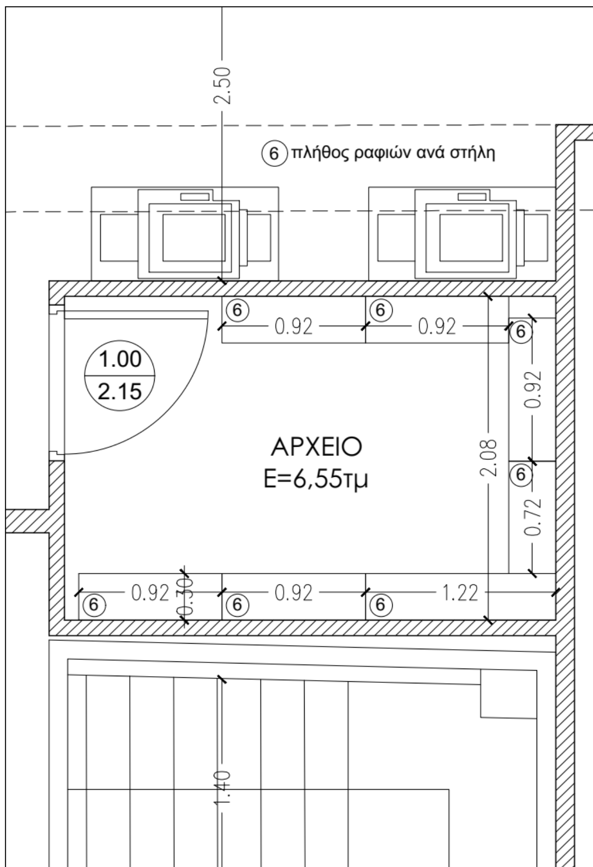
Εικόνα 4. Διάταξη ραφιών αρχειοθέτησης τύπου dexion σε χώρο αρχείου του 2 ου ορόφου.
