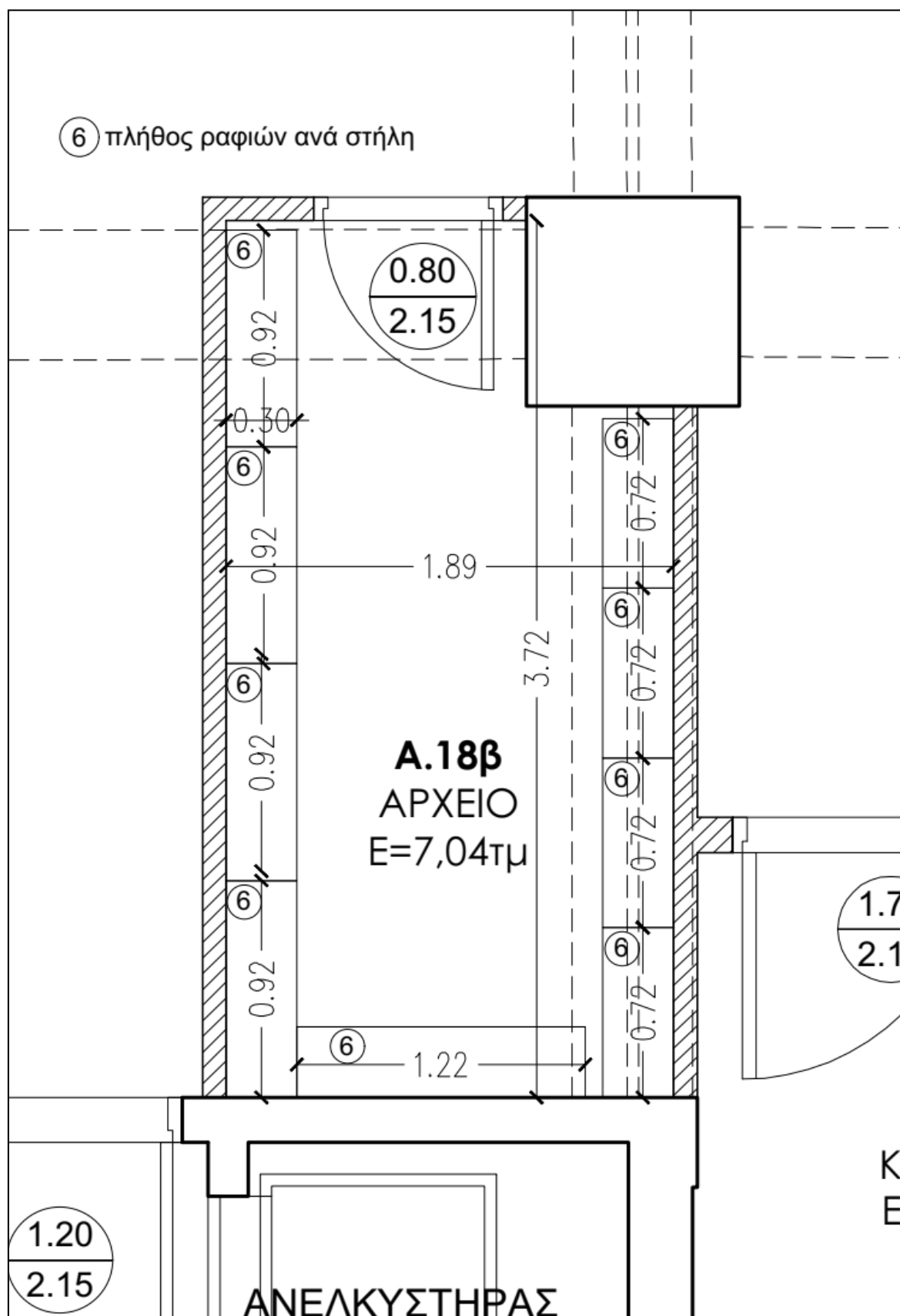
Εικόνα 3. Διάταξη ραφιών αρχειοθέτησης τύπου dexion σε χώρο αρχείου του 1 ου ορόφου.
