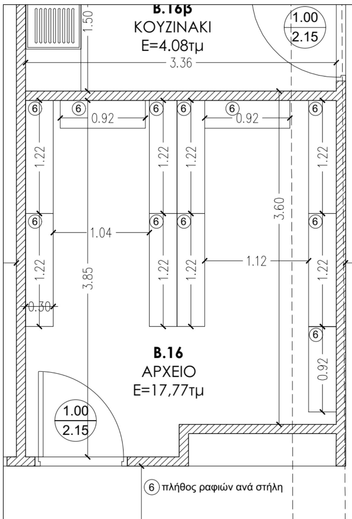
Εικόνα 5. Διάταξη ραφιών αρχειοθέτησης τύπου dexion σε χώρο αρχείου του 2 ου ορόφου.
