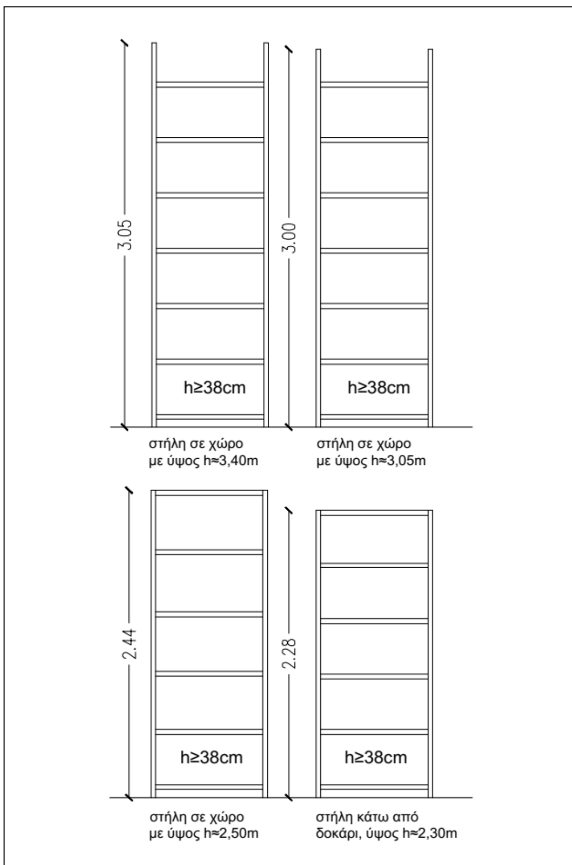
Εικόνα 9. Στήλες ραφιών αρχειοθέτησης τύπου dexion.
