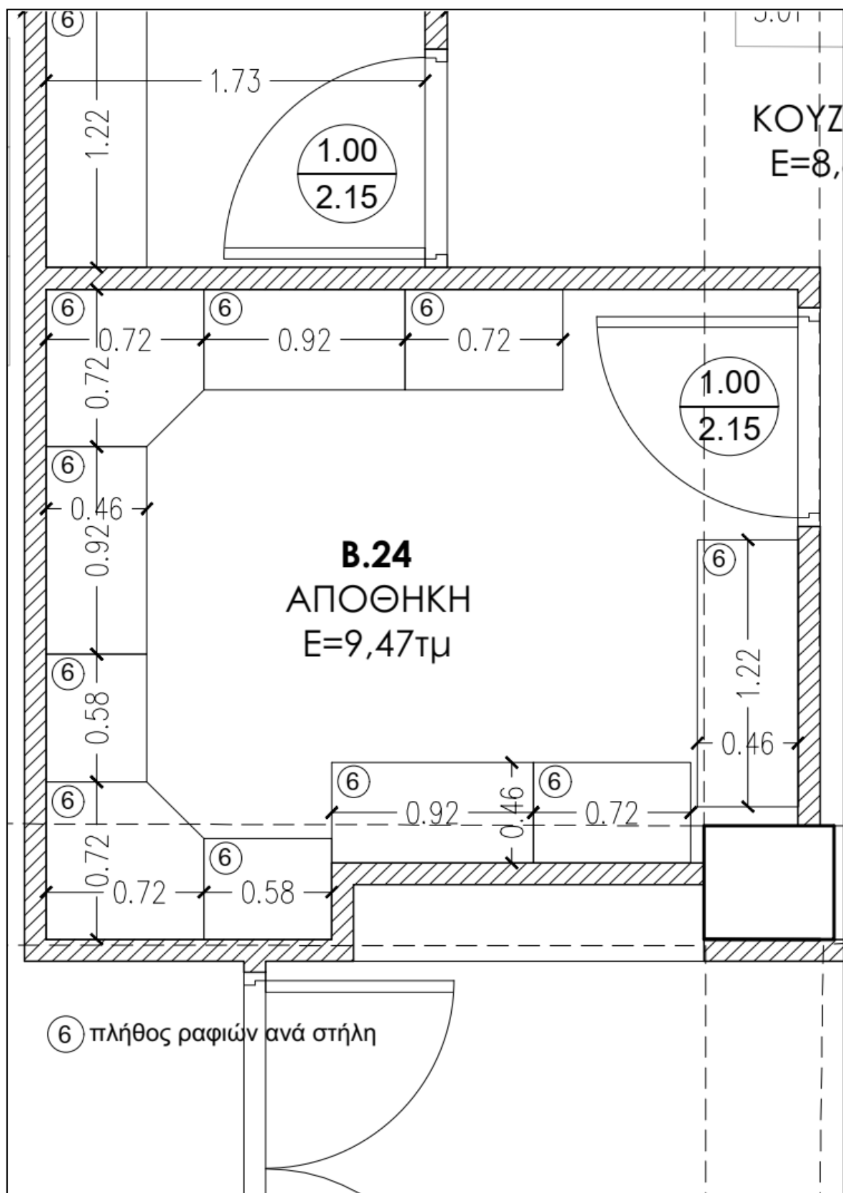
Εικόνα 6. Διάταξη συστήματος ραφιών τύπου dexion σε αποθηκευτικό χώρο του 2 ου ορόφου.
