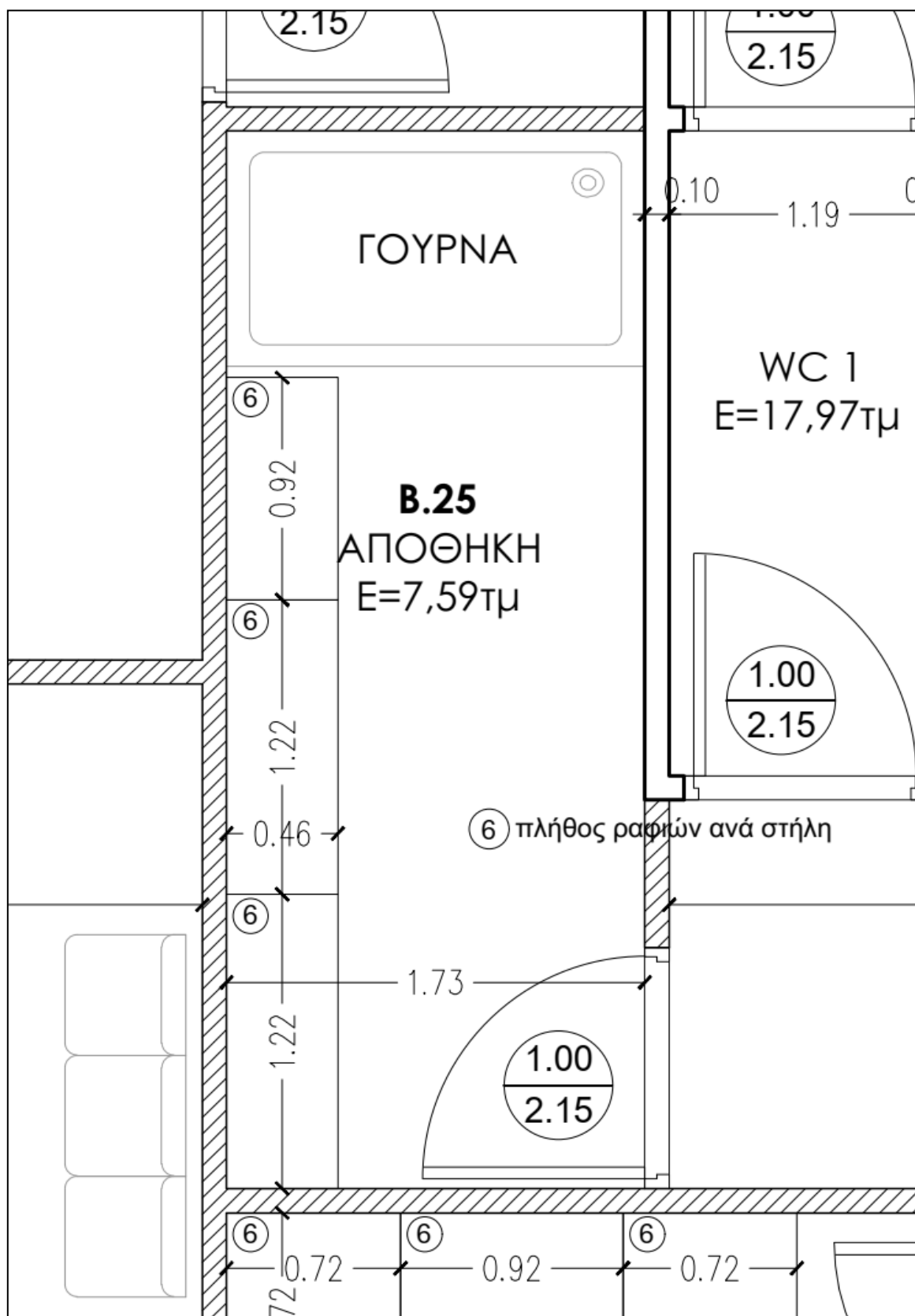
Εικόνα 7. Διάταξη συστήματος ραφιών τύπου dexion σε αποθηκευτικό χώρο του 2 ου ορόφου.
