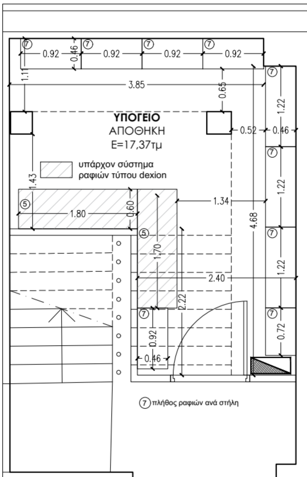
Εικόνα 8. Διάταξη συστήματος ραφιών τύπου dexion σε αποθηκευτικό χώρο του υπογείου.
