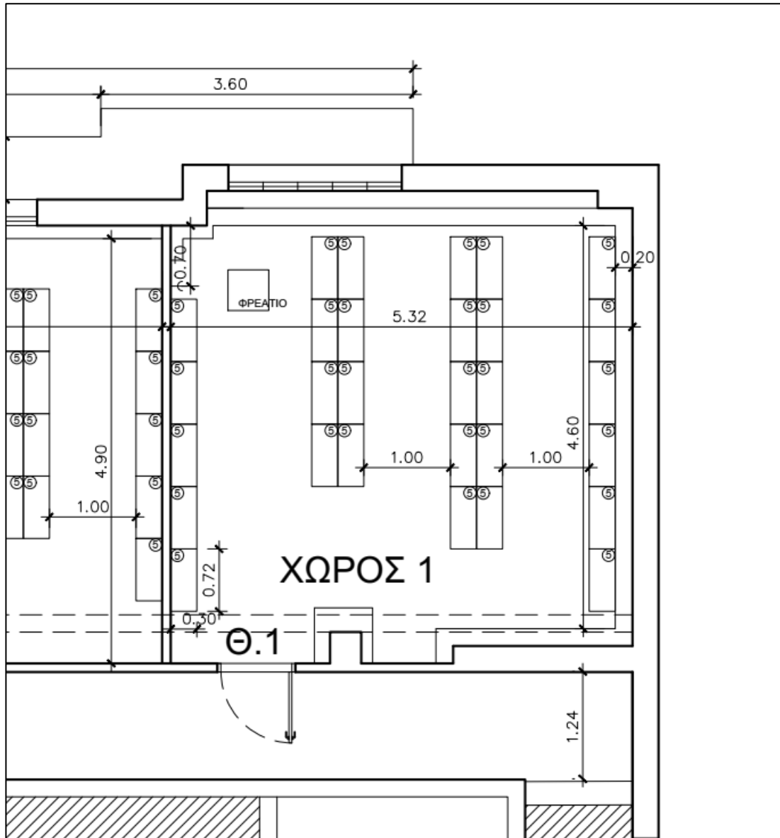
Σχέδιο 1. Διάταξη ραφιών αρχειοθέτησης τύπου dexion στον υπόγειο Χώρο 1.
