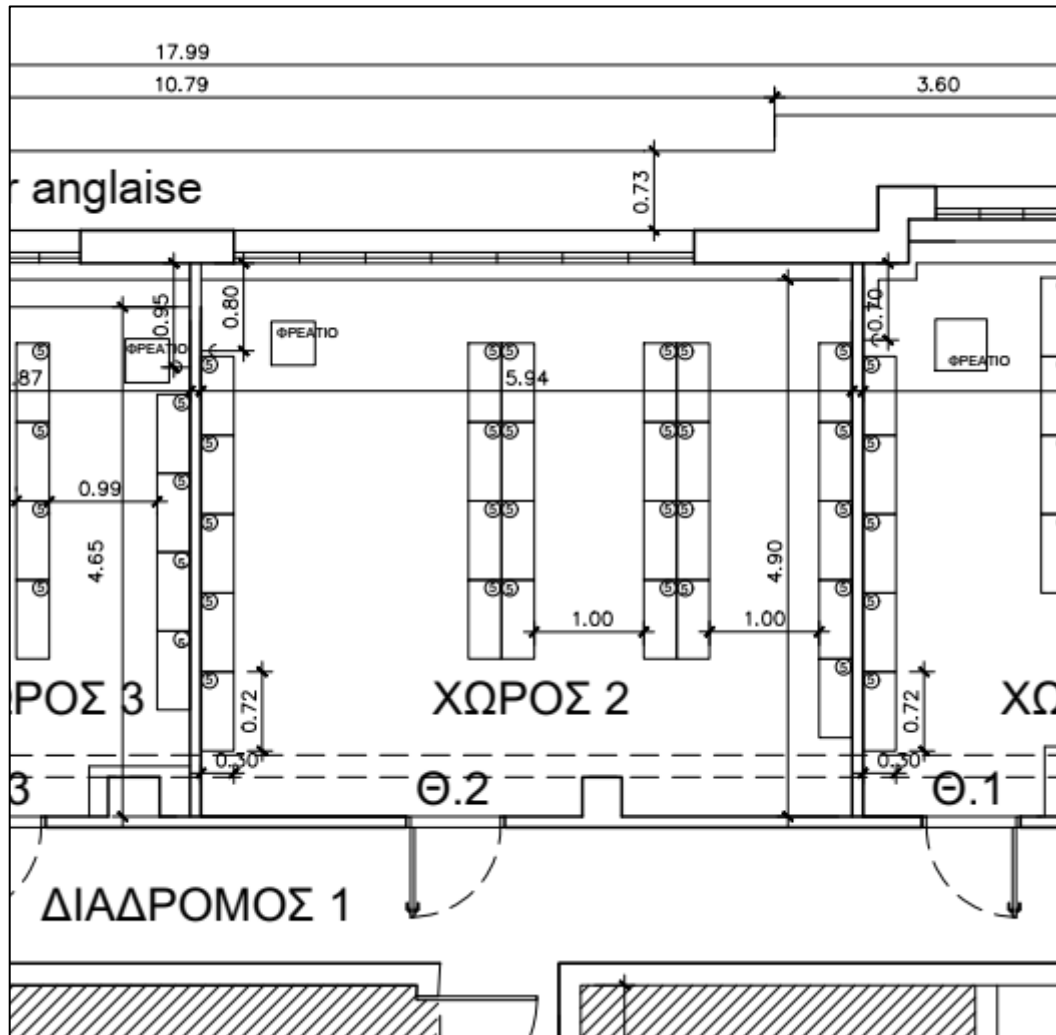
Σχέδιο 2. Διάταξη ραφιών αρχειοθέτησης τύπου dexion στον υπόγειο Χώρο 2.
