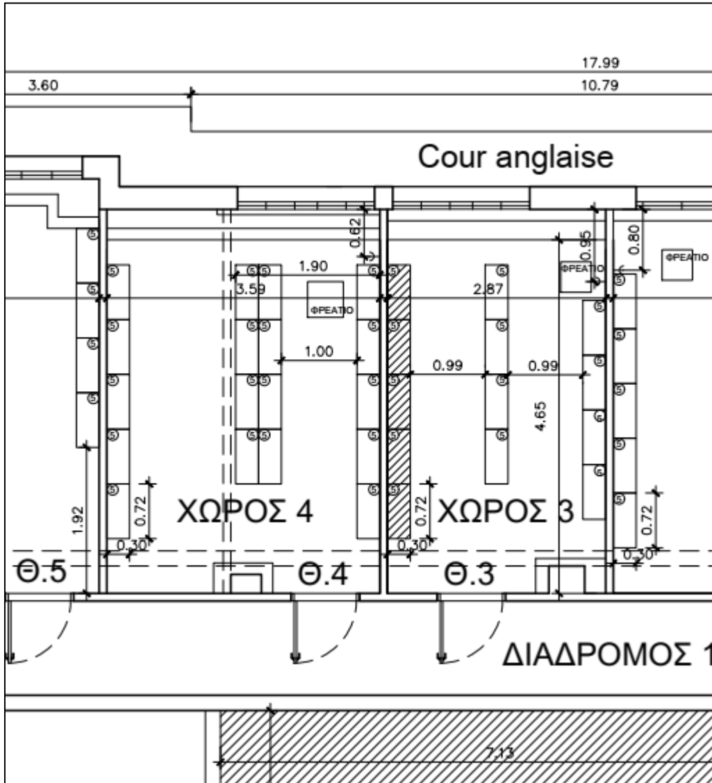
Σχέδιο 3. Διάταξη ραφιών αρχειοθέτησης τύπου dexion στους υπόγειους Χώρους 3 και 4.
