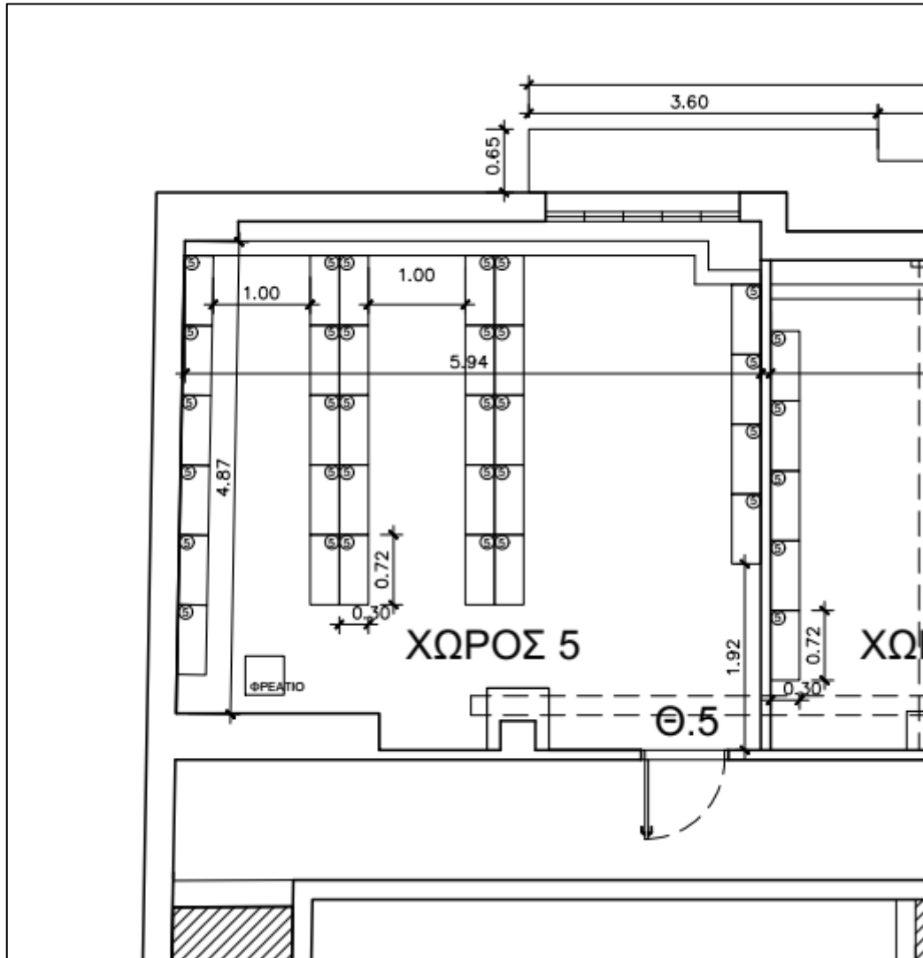
Σχέδιο 4. Διάταξη ραφιών αρχειοθέτησης τύπου dexion στον υπόγειο Χώρο 5.
