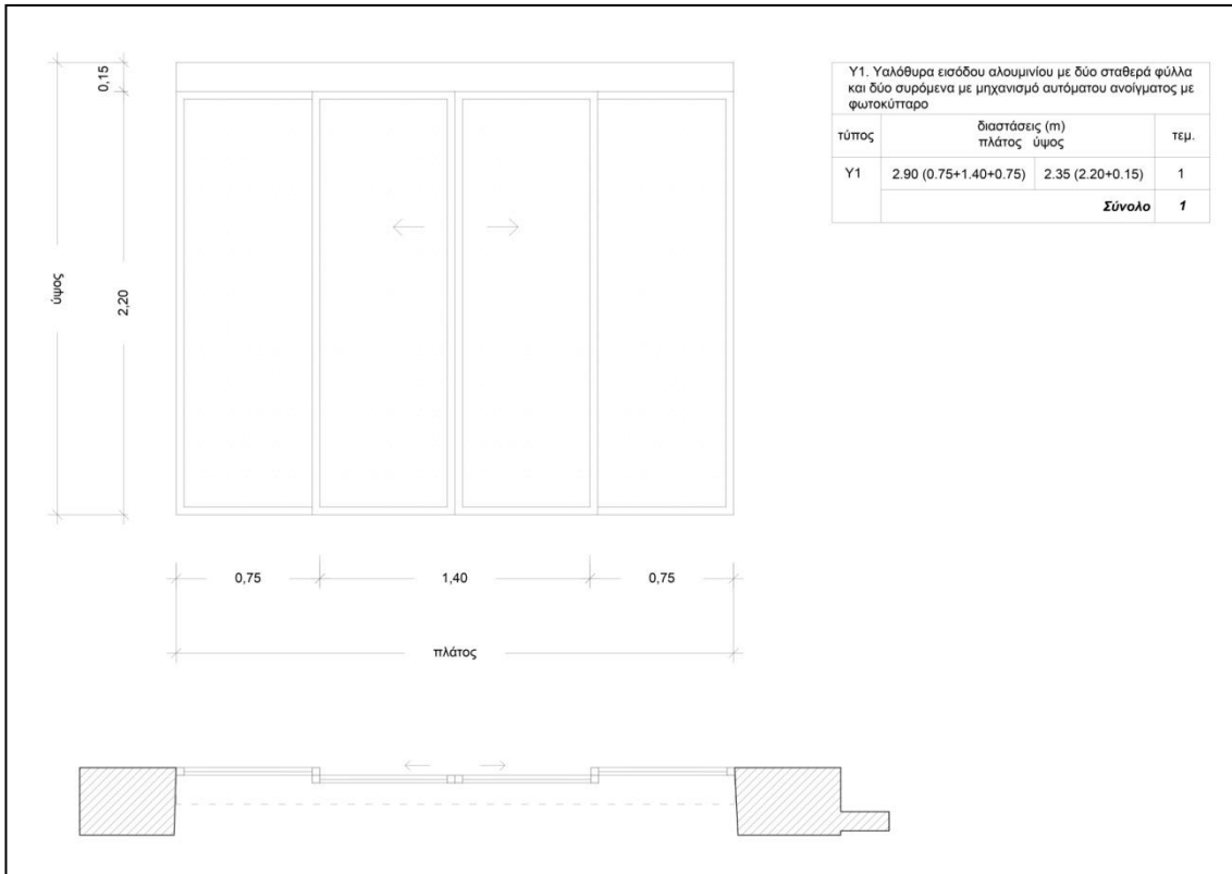
Εικόνα 1. Όψη & κάτοψη νέας αυτόματης υαλόθυρας (Y1) στο Κ.Υ. Ξάνθης
