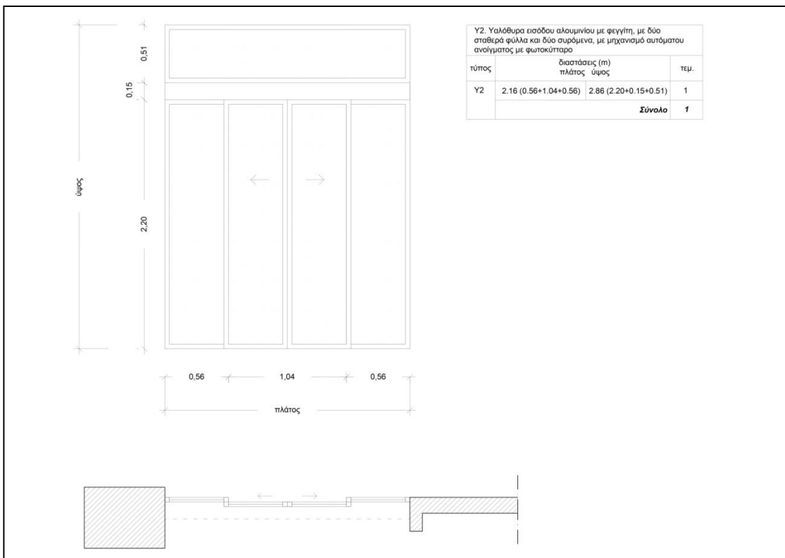
Εικόνα 2. Όψη & κάτοψη νέας αυτόματης υαλόθυρας (Y2) στο Κ.Υ. Ξάνθης
